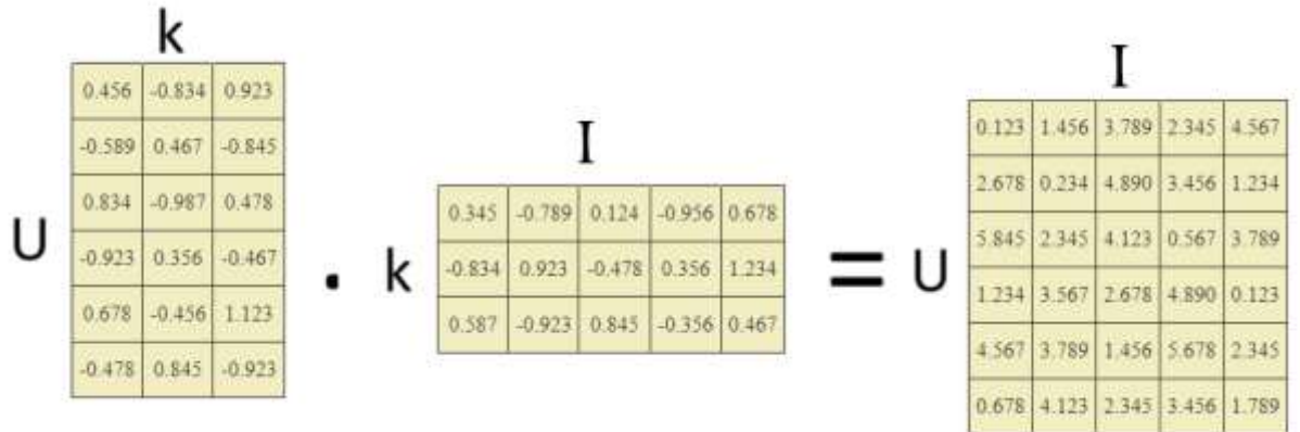
Fig. 2. Latent matrixes after ALS (Matrix factorization).
