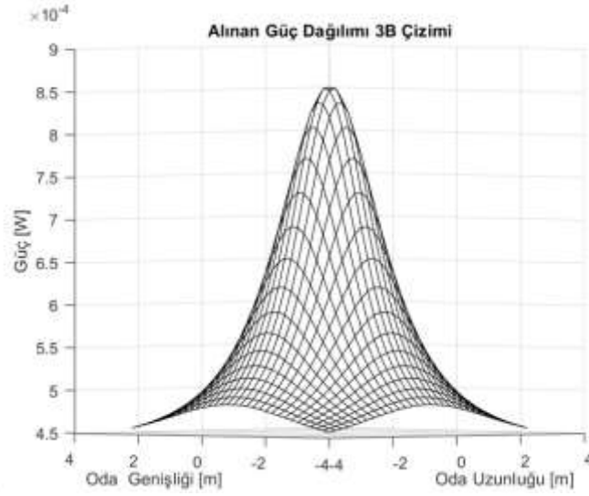
Şekil 3. Tablo 2’deki parametrelerle merkeze yerleştirilmiş bir verici olduğu durumda odadaki alınan güç dağılımı
