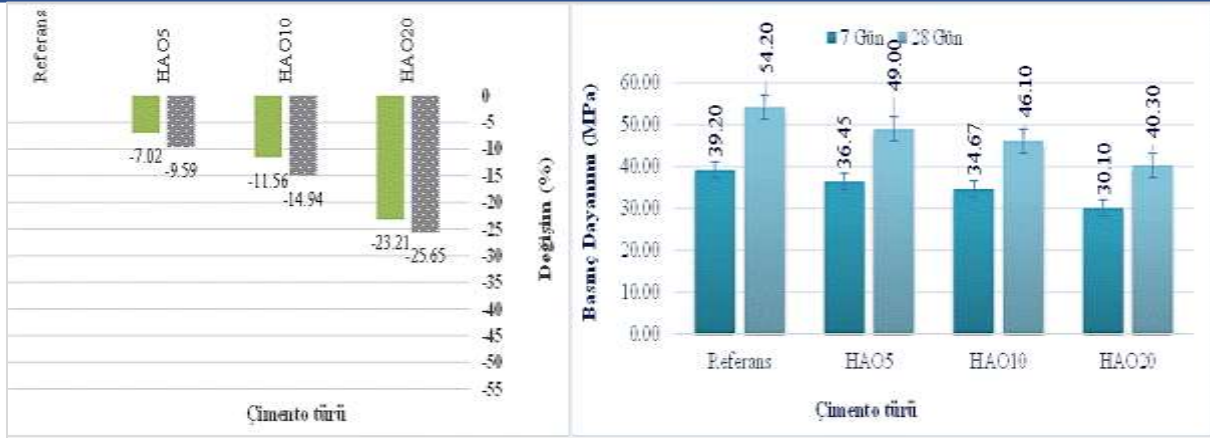
Şekil 6. Test edilen çimentoların referans örneğe göre değişimleri (%) ve basınç dayanımları (MPa)
