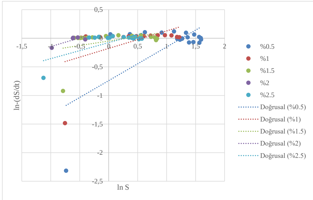
Şekil 10. Şişme Hızının Nümerik Metod ile Bulunması
