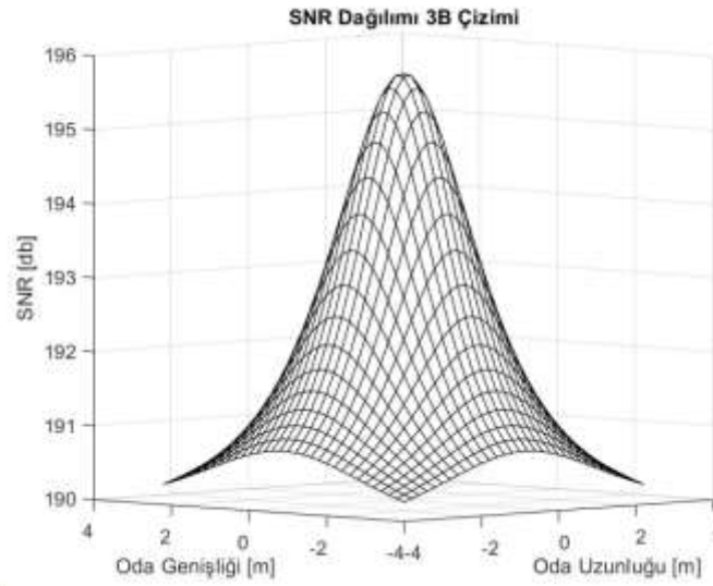
Şekil 5. Tablo 2’deki parametrelerle merkeze yerleştirilmiş bir verici olduğu durumda sinyal gürültü oranı (SNR) dağılımı gösterimi Her üç şekilde de görülebileceği üzere, bir ışık vericisinin merkezde bulunduğu durumda alıcıya en yüksek güçte sinyal iletebileceği aralık, yine merkezde yer alan doğrudan görüş (LOS) bölgeleridir.
