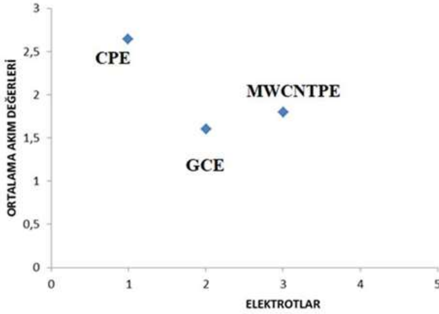
Şekil 2. Pirfenidon tayini için farklı elektrotlar kullanılarak DP voltametri ile elde edilen elektrot-akım değeri grafiğı
