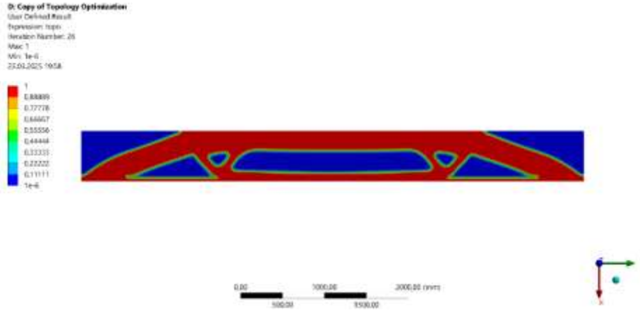
Şekil 4. Topoloji optimizasyonu yoğunluk haritası
