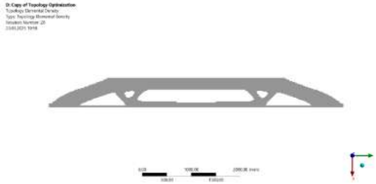
Şekil 3. Çubuk benzeşimi yöntemi sonrası efektif alan görünüşü
