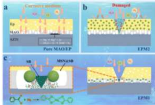
Şekil 2.7. Nanokonteynerlerin konumlarının kaplamanın korozyon koruma performansını arttırması için önerilen koruyucu mekanizma (Zhang, Liu, Sui, Sun, Cui, Kannan, & Zeng, 2023).
