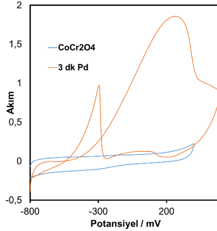
Şekil 2.3. Pd-CoCr 2 O 4 ve CoCr 2 O 4 elektrotlarda etanol oksidasyonu için kaydedilen CV grafikleri
