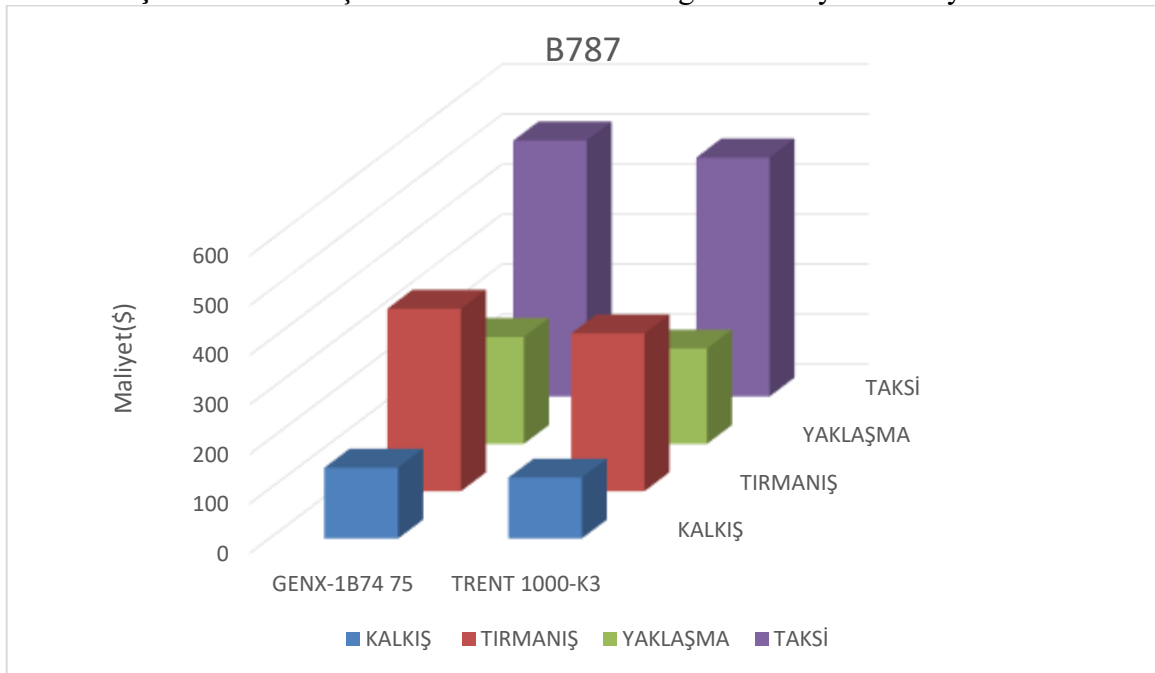
Şekil 4. B787 uçak motorlarının LTO döngüsündeki yakıt maliyetleri
