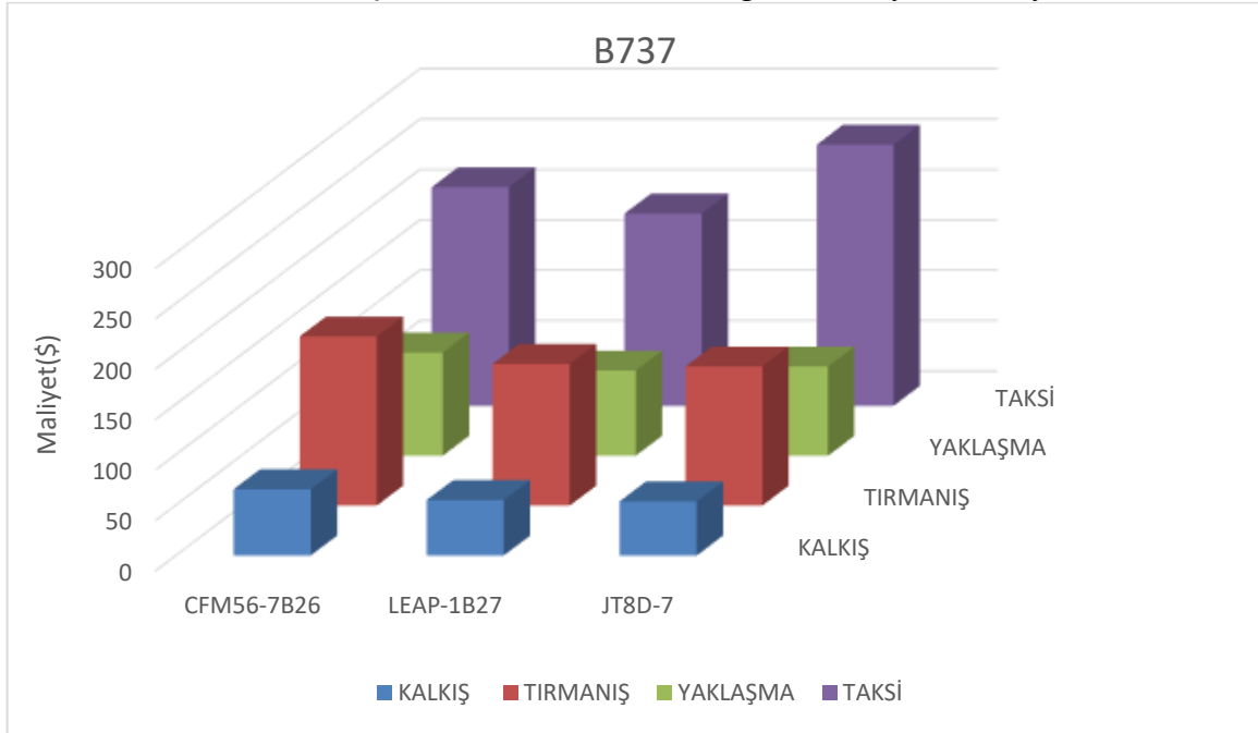
Şekil 2. B737 uçak motorlarının LTO döngüsündeki yakıt maliyetleri
