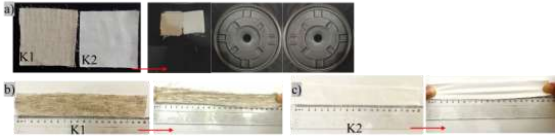
Şek 2. a) Buruşma dayanımı testi uygulaması b) Esneme ve toparlama testi uygulaması
