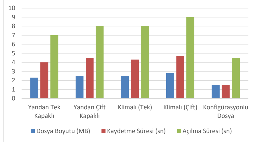
Şekil 7 : Konfigürasyonlara göre dosyaların performans kıyaslaması.
