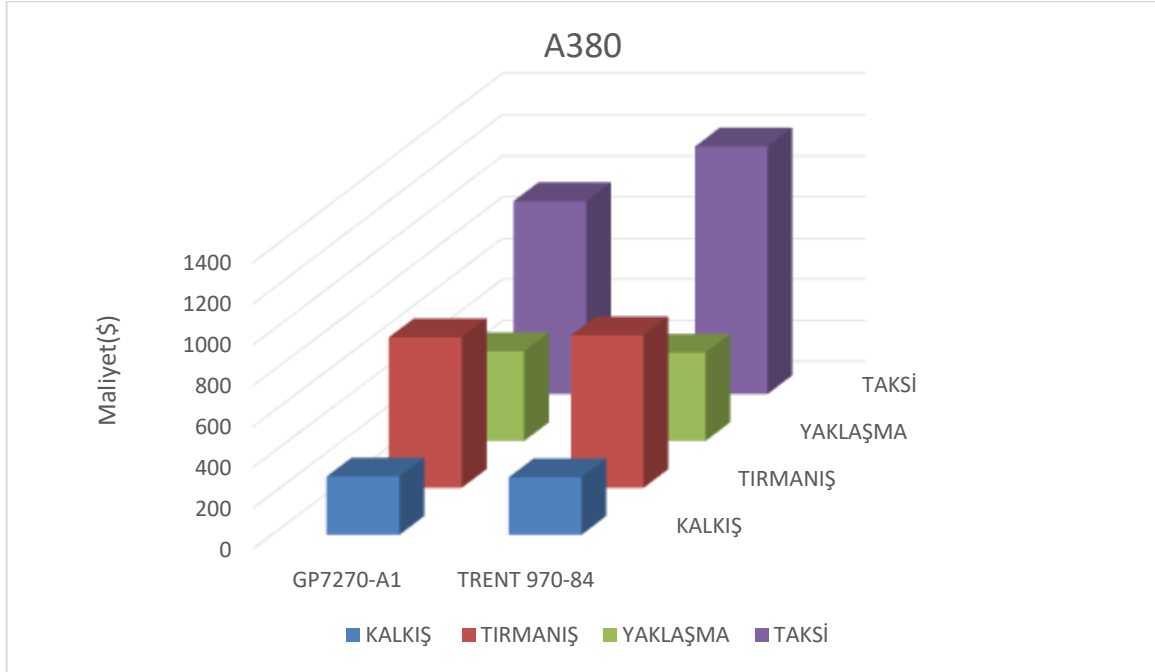
Şekil 3. A380 uçak motorlarının LTO döngüsündeki yakıt maliyetleri
