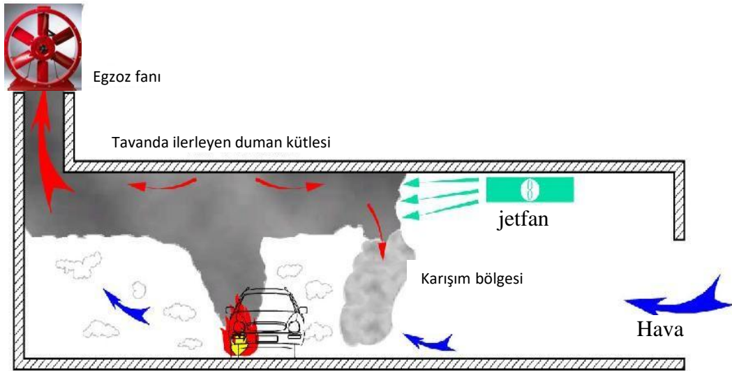
Resim 3.Jet fun Sistemi
