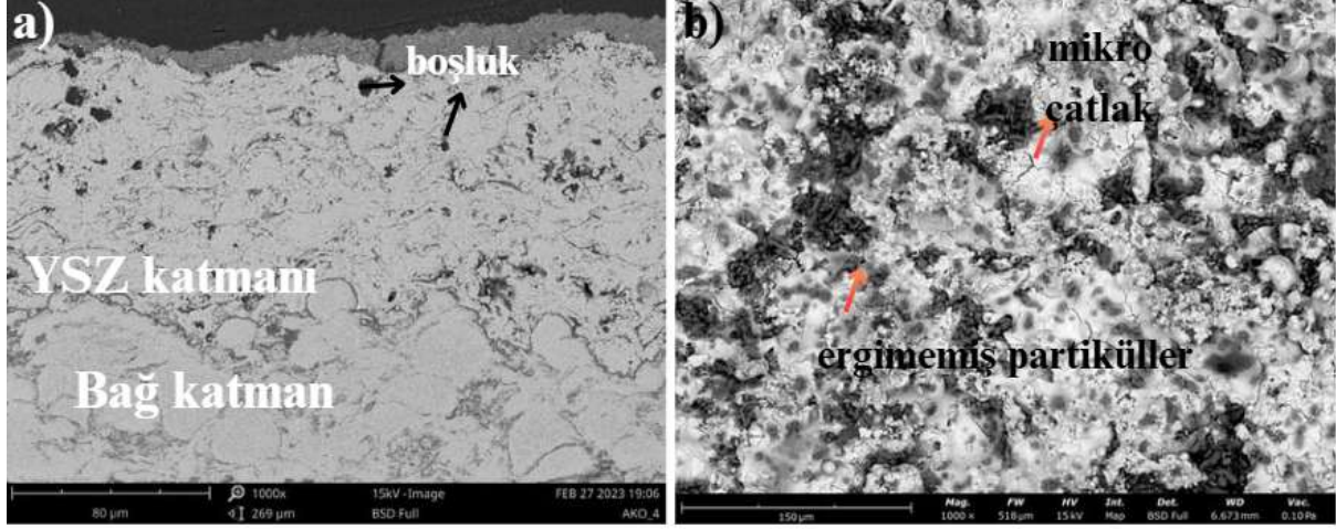
Şekil 4. YSZ kaplamanın SEM resimleri: a) Kesit, b) Yüzey
