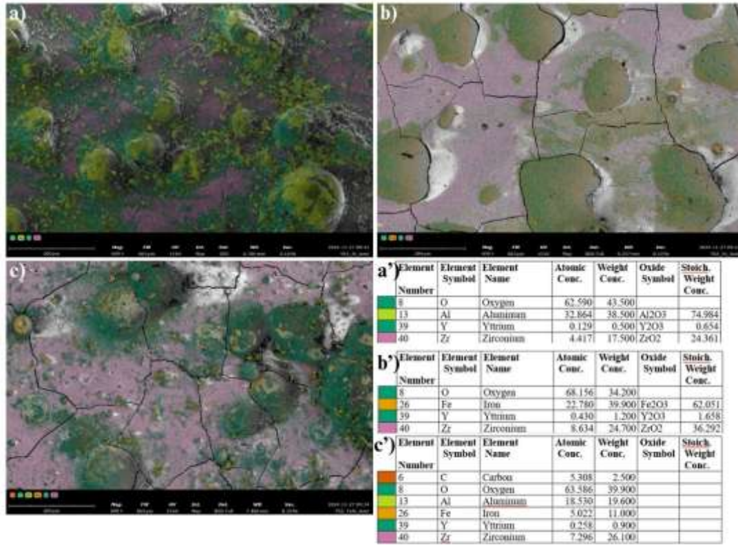
Şekil 5. SEM resimleri: a) Al tozu tatbik edilmiş numune, b) Fe tozu tatbik edilmiş numune, c)
