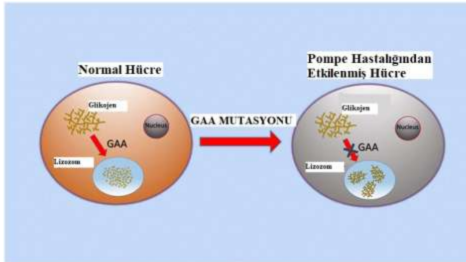
Şekil 1. PH hücrelerinin lizozomlarında glikojen depolanmasına neden olan GAA değişikliğinin şematik gösterimi (Taverna vd., 2020).
