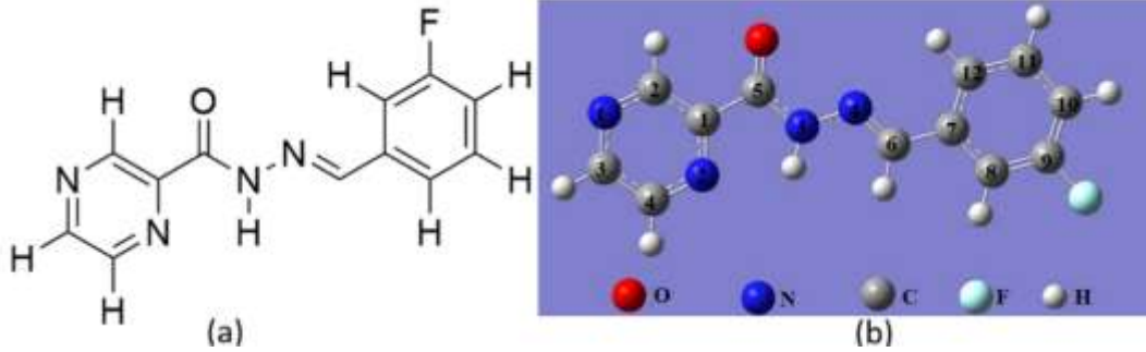
Şekil 1. Molekülün, kimyasal yapısı ve numaralandırılmış optimize durumu
