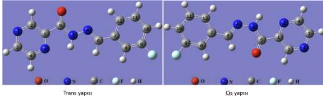
Şekil 3. Molekölün optimize şekli
