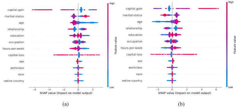
Şekil 3.3. SHAP Algoritmasının Parametrelerin Sınıflara Etki Grafiği
