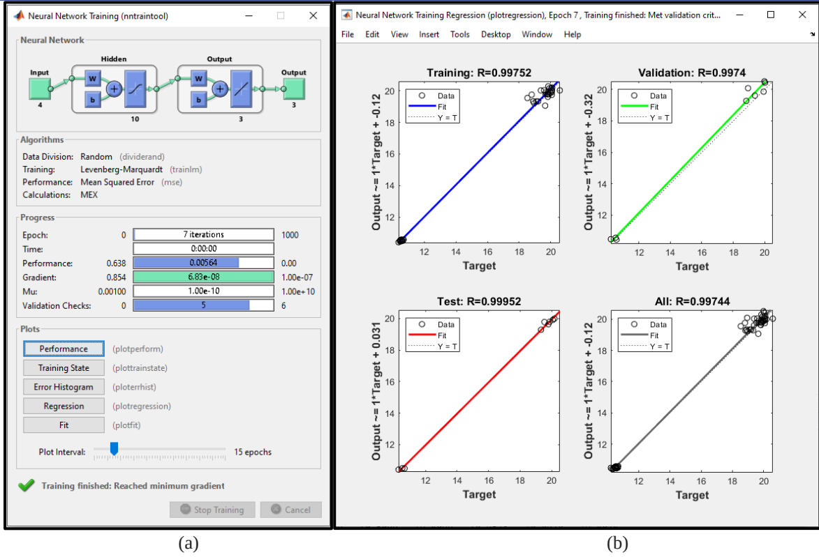
Şekil 3. (a) Çok katmanlı algılayıcı sinir ağının uygulanması ve (b) verilerin regresyon diyagramı.
